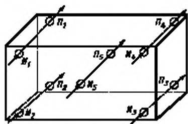
N_1, N_2, N_3, N_4, N_5 — точки установки излучающего электроакустического преобразователя; N_6, N_7, N_8, N_9, N_{10}, N_{11}, N_{12}, N_{13}, N_{14}, N_{15}, N_{16}, N_{17} — точки установки приемного электроакустического преобразователя
