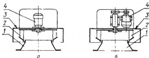
1 - входной патрубок; 2 - рабочее колесо; 3 - корпус; 4 - электродвигатель
