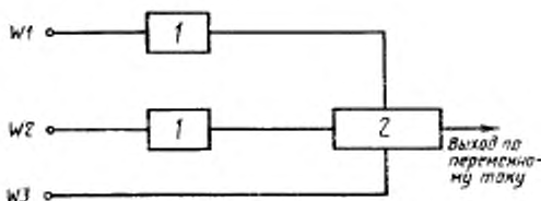
1 — единица СБП; 2 — переключающее устройство
