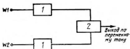
W1, W2 — входы по переменному току; 1 — единица СБП; 2 — переключающее устройство
