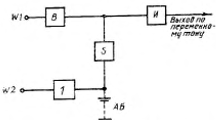
Цепь постоянного тока
