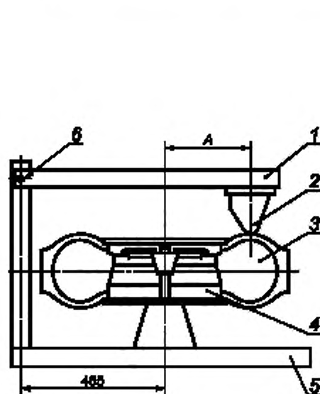
1 — подвижный рычаг; 2 — специальный упор; 3 — шина; 4 — обод; 5 — неподвижная плита (основание); 6 — ось поворота рычага
