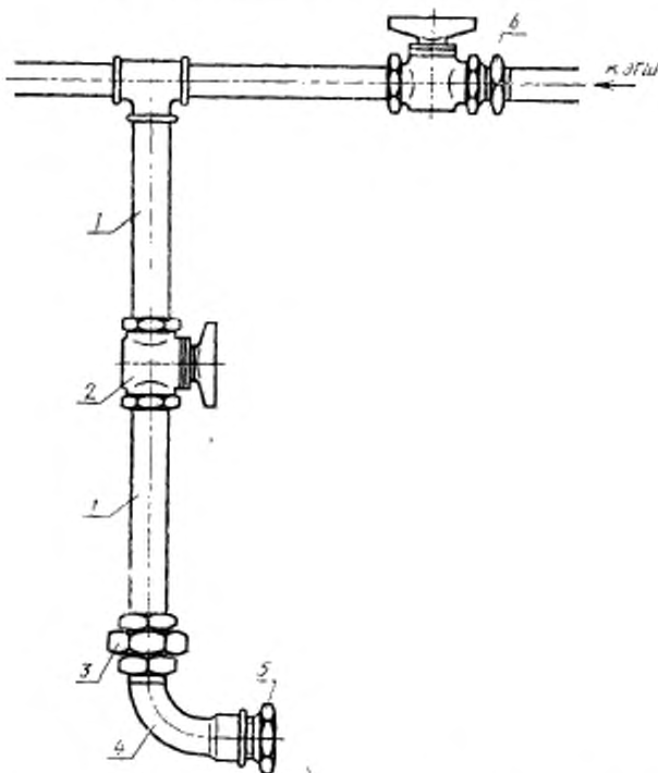
Схема присоединения однопроводного клапана
