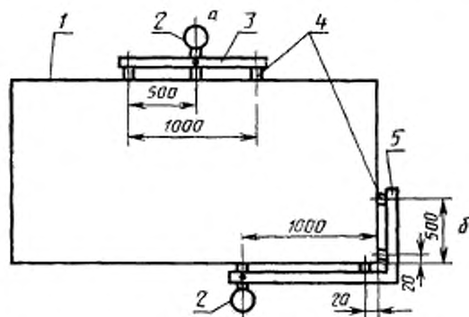
Схема измерения прямолинейности и перпендикулярности кромок
