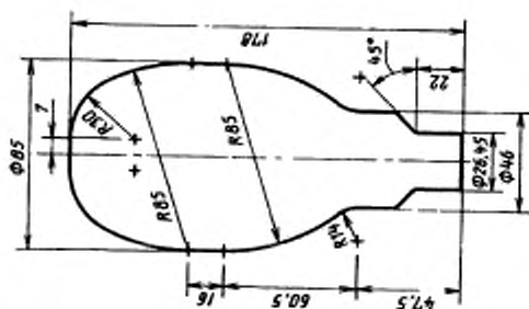
Наибольший контур ртутной лампы высокого давления мощностью 125 Вт
