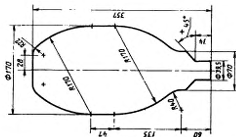
Наибольший контур ртутной лампы высокого давления мощностью 700 Вт с цоколем E40
