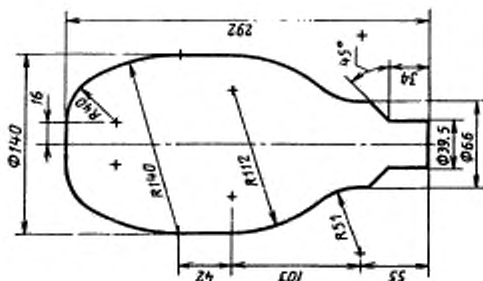
Наибольший контур ртутной лампы высокого давления мощностью 400 Вт
