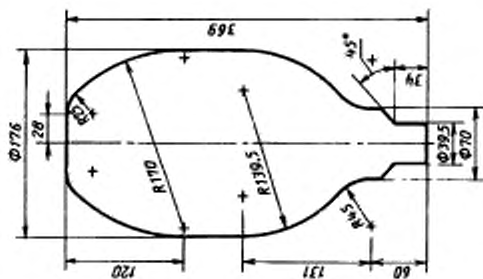
Наибольший контур ртутной лампы высокого давления мощностью 700 Вт с цоколем E39
