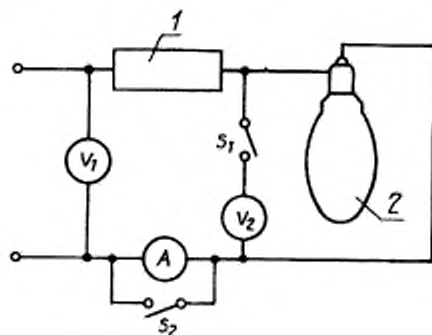
1 — балласт, 2 — лампа
