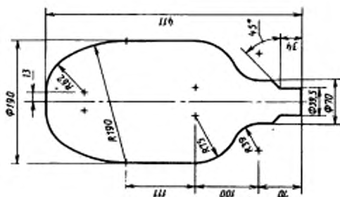
Наибольший контур ртутной лампы высокого давления мощностью 1000 Вт с цоколем E40
