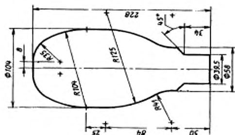
Наибольший контур ртутной лампы высокого давления мощностью 175 и 250 Вт
