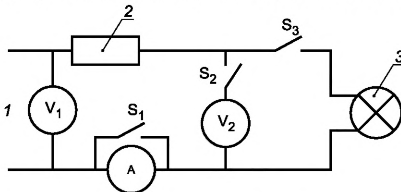
1 — источник питания; 2 — эталонный балласт; 3 — лампа
