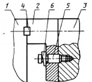
1 — монтажная плита; 2 — монтажный мостик; 3 — кокиль; 4 — шпонка; 5 — штифт; 6 — клин
