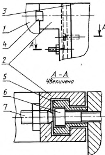
1 — монтажная плита; 2 — монтажный мостик; 3 — кокиль; 4 — шпонка; 5 — Т-образная шпонка; 6 — винт; 7 — распорный винт
