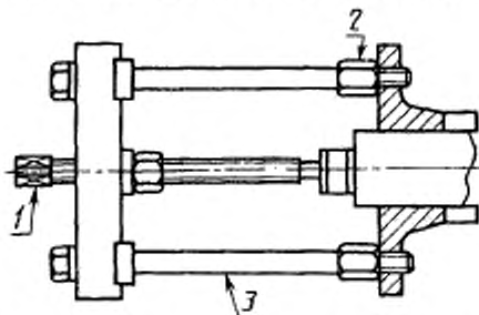
А. 2. Съемник с резьбовым присоединением (черт. 10)
