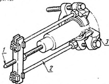
А. 4. Съёмник с приспособлением для наружного захвата (черт. 12)
