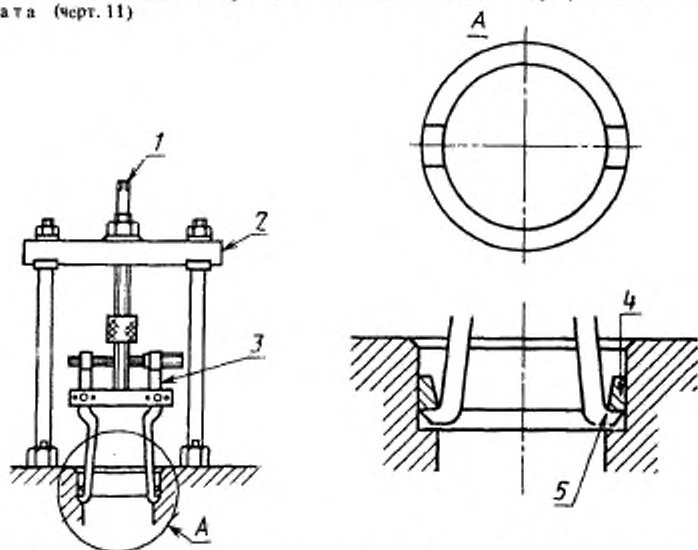
А. 3. Съёмник с приспособлением для внутреннего захвата (черт. 11)
