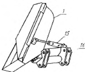
1—ковш; 15—гидроцилиндр боковой разгрузки; 16—рама ковша с люлькой
