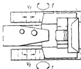
Черт. 11. С независимым вращением двигателей каждого борта, v_1 \neq v_2 (гусеничный погрузчик)
