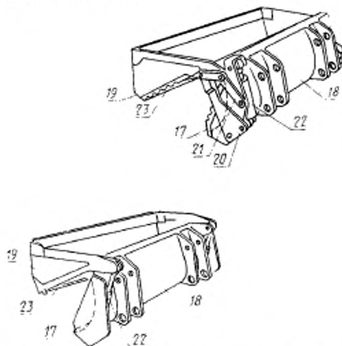
17—режущая кромка бульдозерной (нижней) челюсти; 18—бульдозерная (нижняя) челюсть; 19—верхняя (подвижная) челюсть; 20—гидроцилиндр; 21—тяга верхней челюсти; 22—гидроцилиндр открывания челюсти; 23—режущая кромка верхней челюсти
