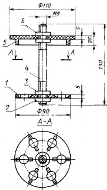
Держатель образцов
