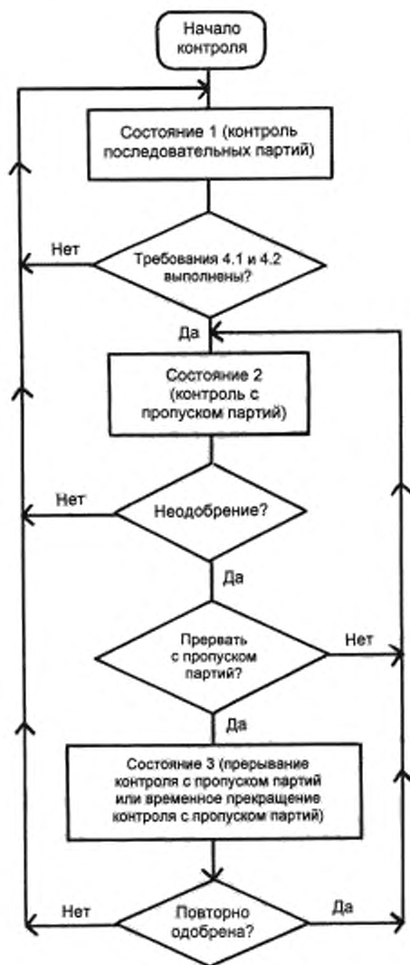
Рисунок 1 — Общая структура процедур с пропуском партий
