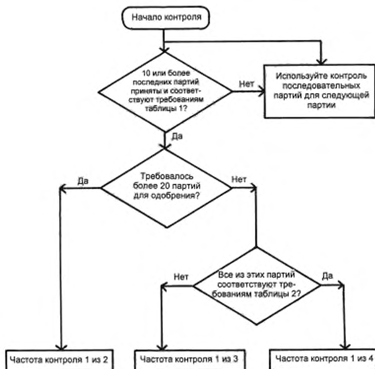
Рисунок 2 — Определение начальной частоты контроля с пропуском партий
