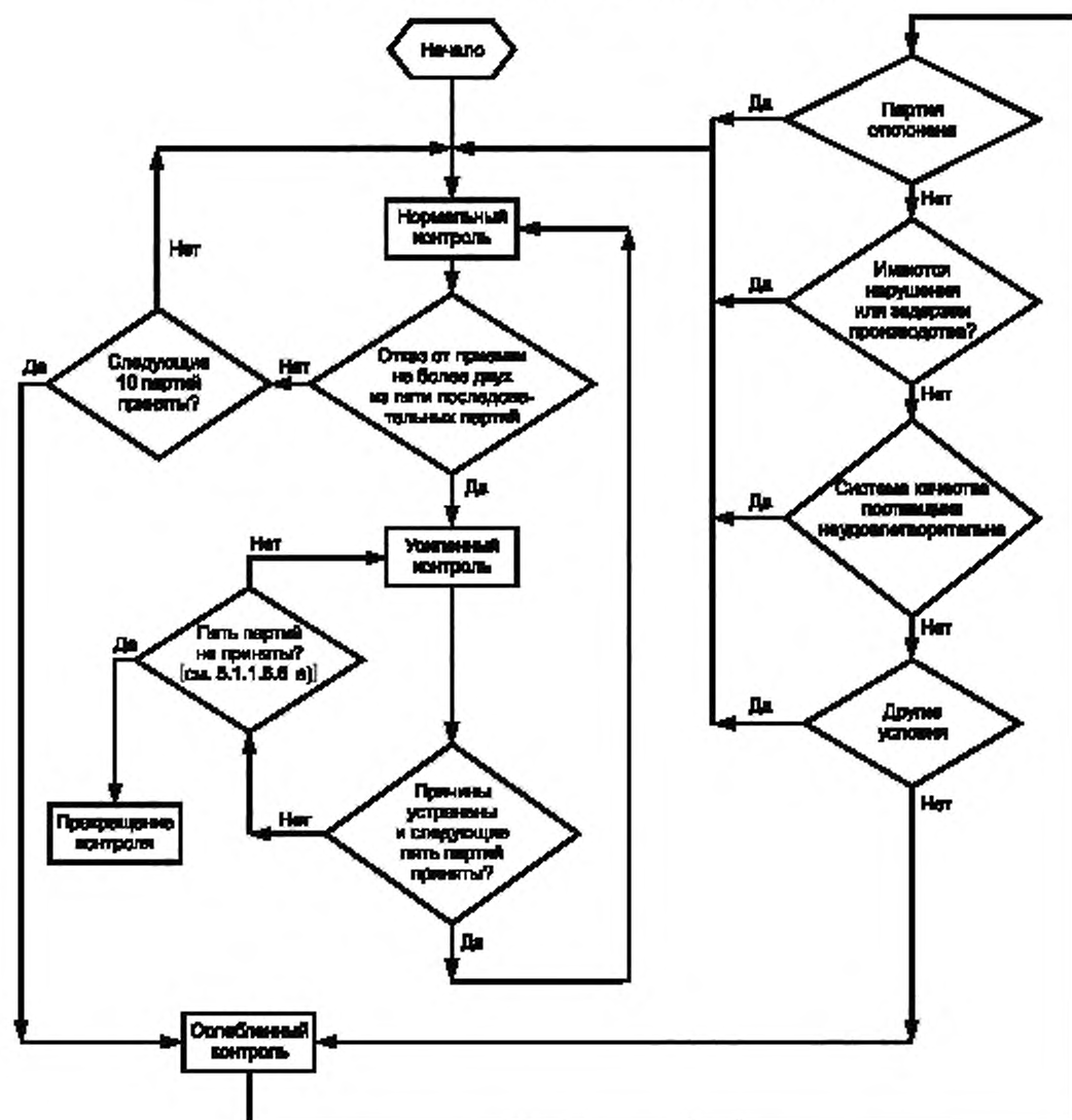
Рисунок С.1 — Процедуры переключения выборочного контроля
