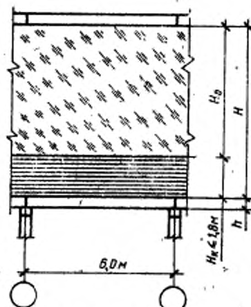
г) с ленточным остеклением
