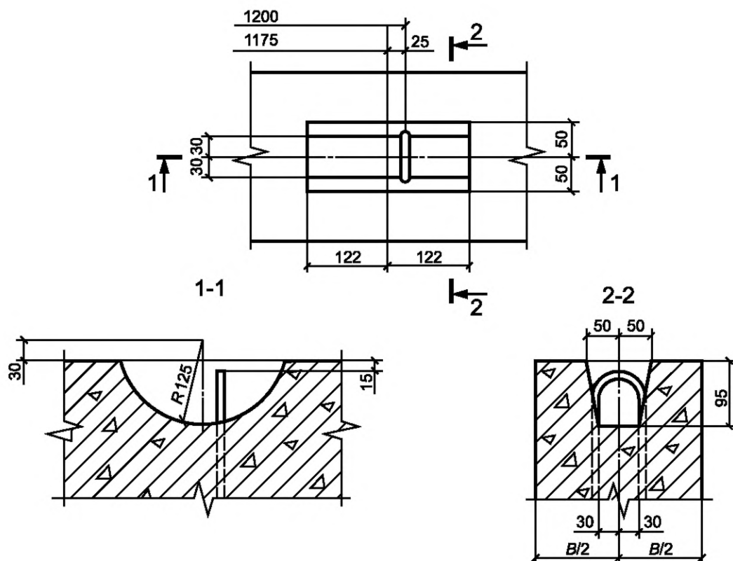
Рисунок 1 — Скрытое расположение монтажной петли
