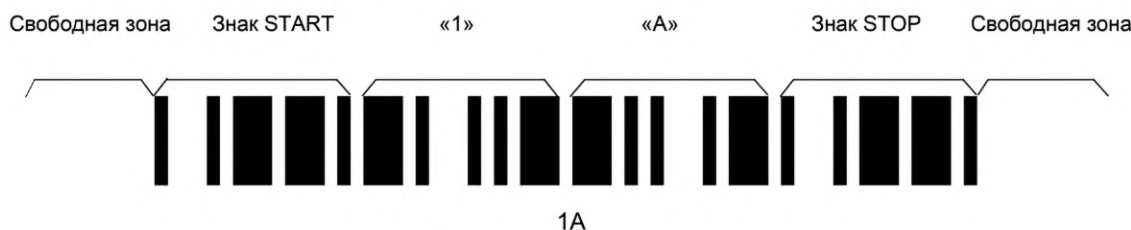
Рисунок 1 — Символ Code 39
