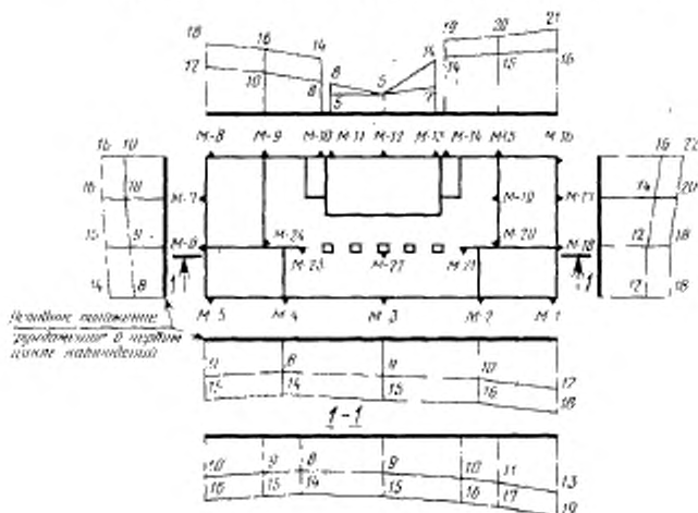
План расположения марок и эпюры перемещений
