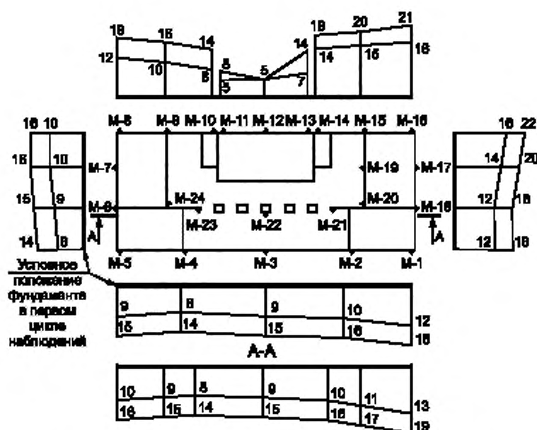
Рисунок Г.2 — План расположения марок и эпюры перемещений
