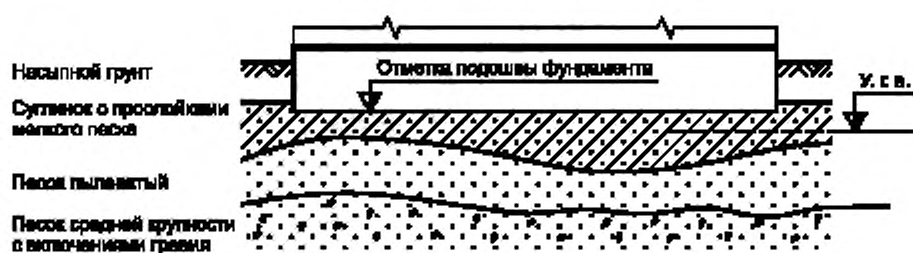
Рисунок Г.1 — Схема фундамента основания
