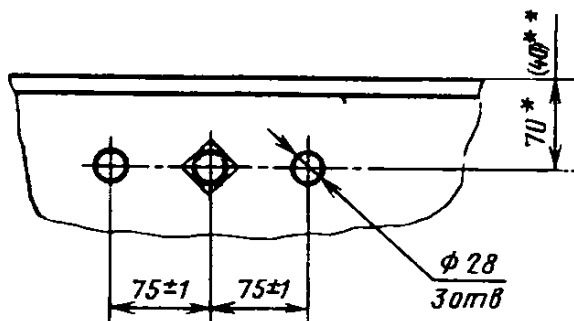
г) для смесителя с нижней камерой смешения
