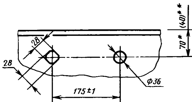
в) для смесителя со шеткой
