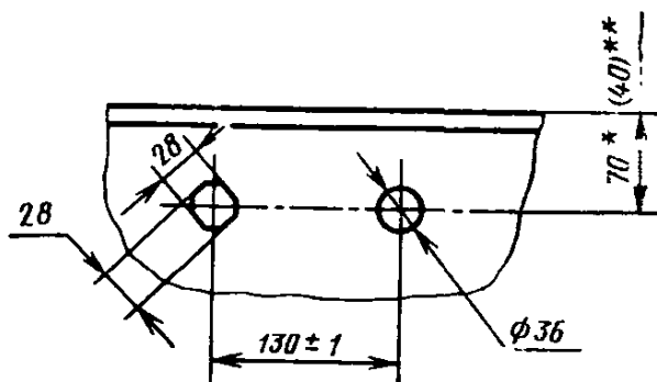
б) для смесителя с одной рукояткой
