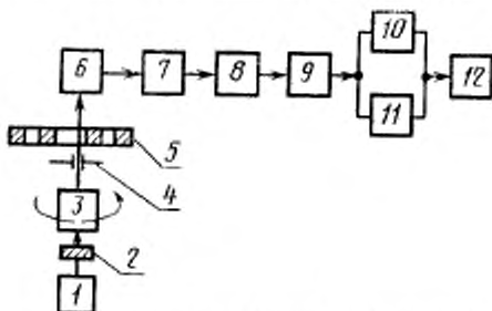
Блок-схема установки для определения ФПМ
