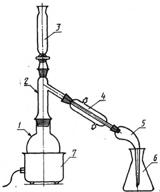
1 — реакционная колба; 2 — переход; 3 — делительная воронка; 4 — холодильник; 5 — шланг; 6 — приемная колба; 7 — электронагревательный прибор
