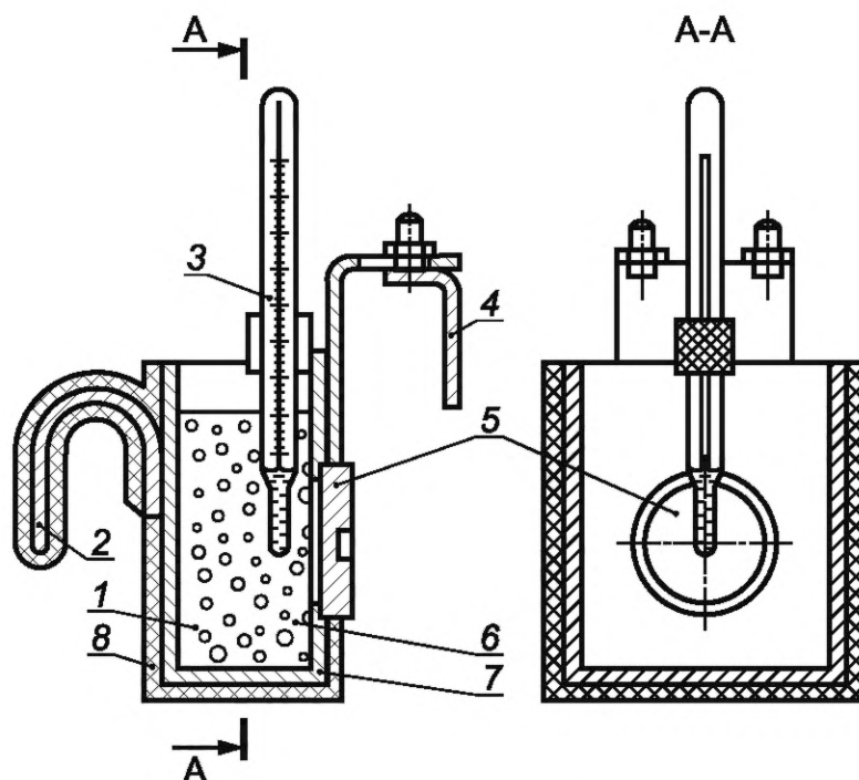
Рисунок 5 — Схема прибора для контроля точки росы
