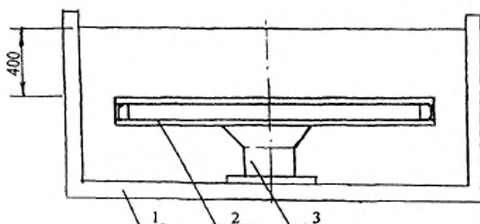
1 — емкость с водой; 2 — образец стеклопакета; 3 — вакуумная присоска
