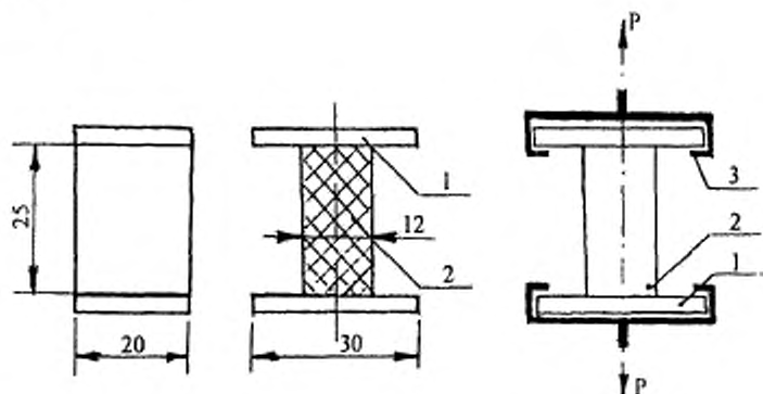
Рисунок 9 — Испытание герметика второго герметизирующего слоя
