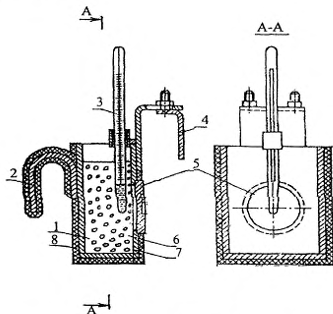
1 — ацетон или изопропиловый спирт; 2 — ручка; 3 — термометр; 4 — подвижная пластина узла подвески; 5 — контактная латунная пластина; 6 — твердая двуокись углерода; 7 — корпус медный; 8 — теплоизоляция
