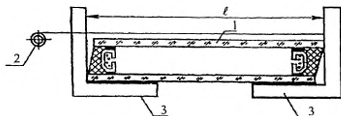
1 — стеклопакет; 2 — рулетка; 3 — угольник, l — контролируемый размер
