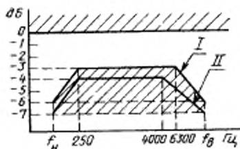
Допускаемая неравномерность амплитудно-частотной характеристики каналов воспроизведения и записи-воспроизведения
