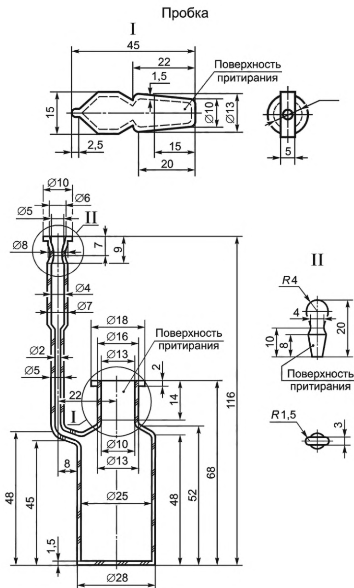
Рисунок 1 — Пикнометры с боковым капилляром вместимостью 20—25 см 3 с хорошо притертыми пробками
