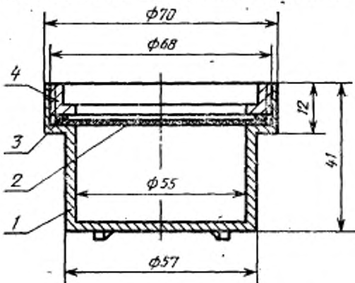
Диффузионная ячейка для гравиметрического метода
