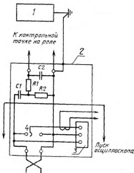
Схема импульсного генератора
