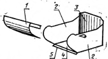
1—заслонка; 2—боковая стенка; 3—подвижная задняя стенка; 4—днище; 5—нож
