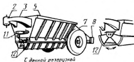
с донной разгрузкой
