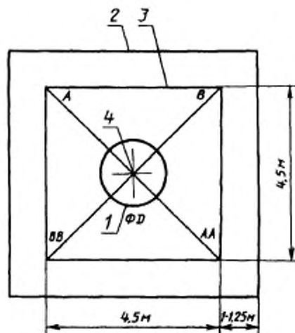
Вид сверху испытательной камеры
