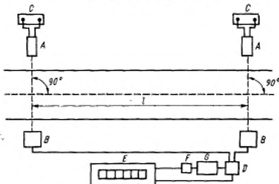
Типовая схема расположения оборудования при измерениях скорости движения машины
