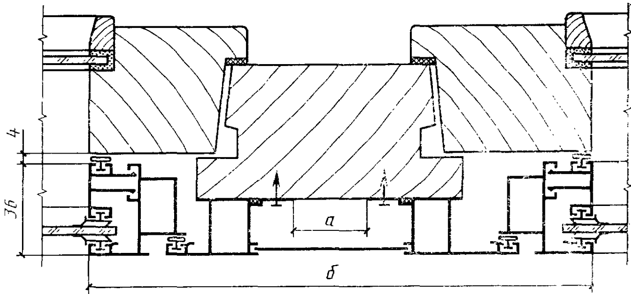
Сечение 5 и 6 (для трехстворчатого окна)
