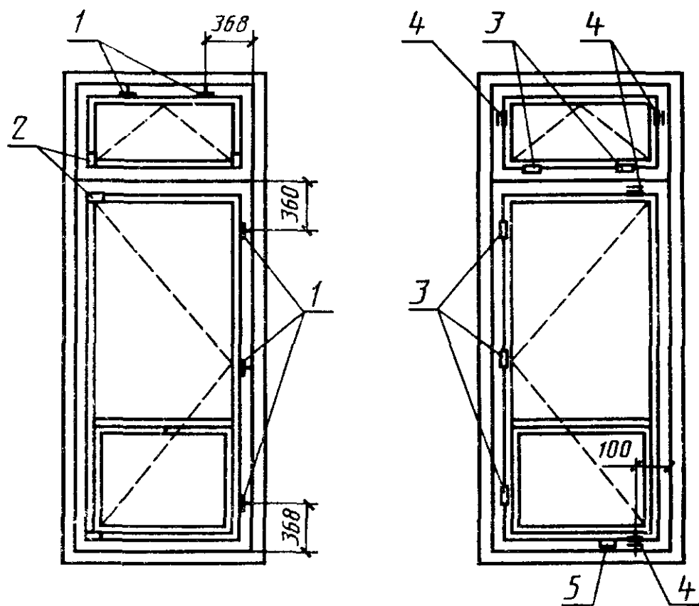
1 — завертка врезная типа ЗР1; 2 — петля для спаривания; 3 — петля; 4 — соединитель створок; 5 — компенсатор
