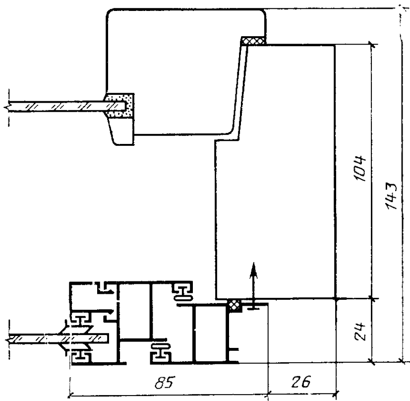
Сечение 4
