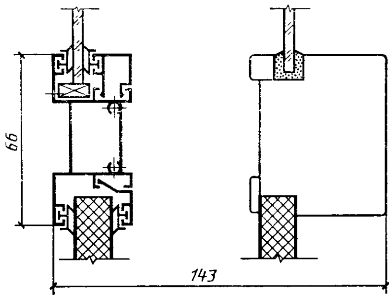
Сечение 7
