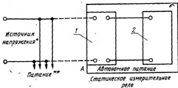
1 — вспомогательный источник реле (входной интерфейс); 2 — статическое реле
