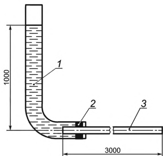
Рисунок 5 — Испытательное устройство
