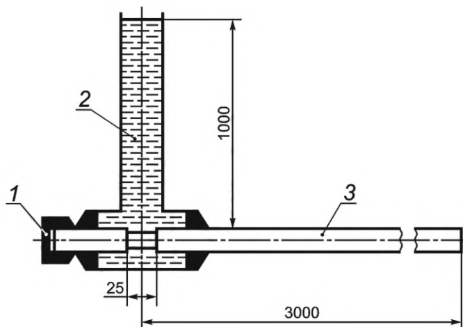
Рисунок 4 — Испытательное устройство
