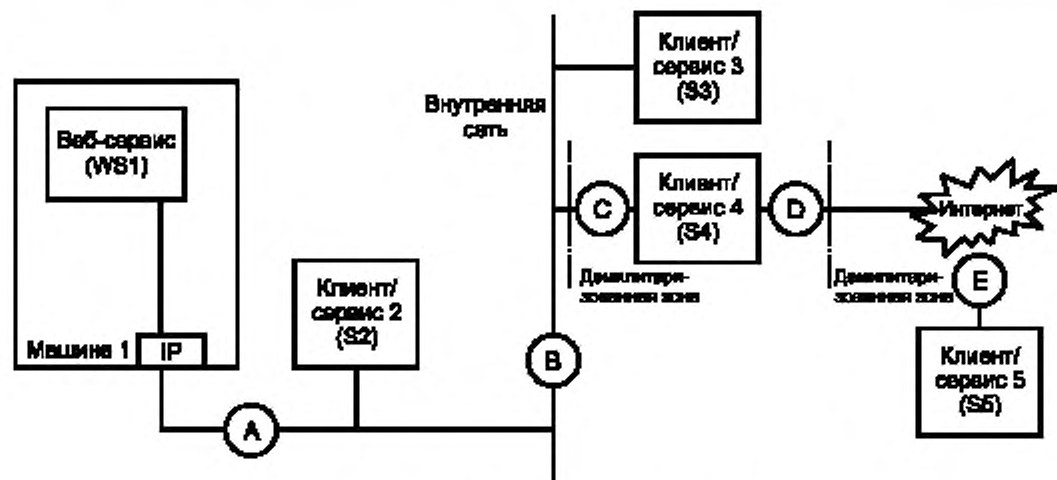
Рисунок В.1 — Общая модель веб-сервисов
