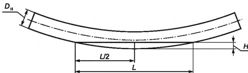
Рисунок 8 — Измерение высоты стрелы прогиба на внутренней поверхности отвода наружным диаметром от 1020 до 1420 мм».
