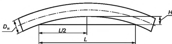
Рисунок 7 — Измерение высоты стрелы прогиба отвода
