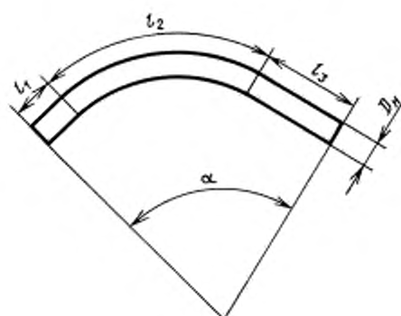
Отвод типа 1
