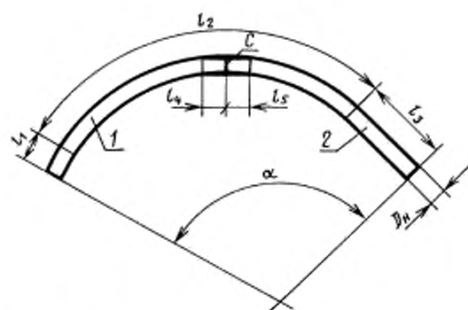
Отвод типа 3
