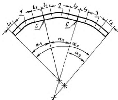
Вставка из трех отводов
