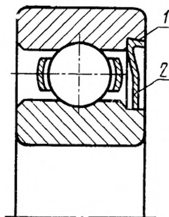
1—канавка под защитную шайбу; 2—защитная шайба
