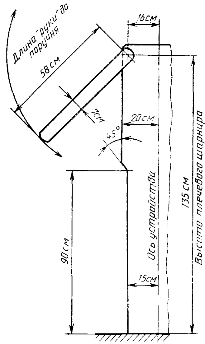
Контрольное устройство для проверки расположения поручней и ручек (см. п. 5.11.2.1)
