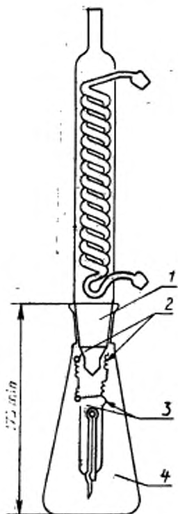
1 — шпиф 34/35; 2 — крючок; 3 — отверстия в экстракционной чашке емкостью 30 см 3 ; 4 — прием. ник емкостью 250 см 3
