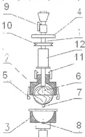
Рисунок А.2 – Механизм отмывания
