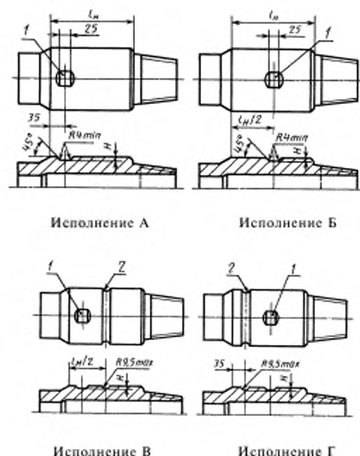
1 — опознавательный паз группы прочности трубы; 2 — опознавательная канавка толщины стенки для группы прочности А и выше; H — глубина опознавательных пазов и канавок: для замков диаметром до 127 мм включительно H = 4,8 мм, для замков диаметром от 133 мм и выше H = 6,4 мм
