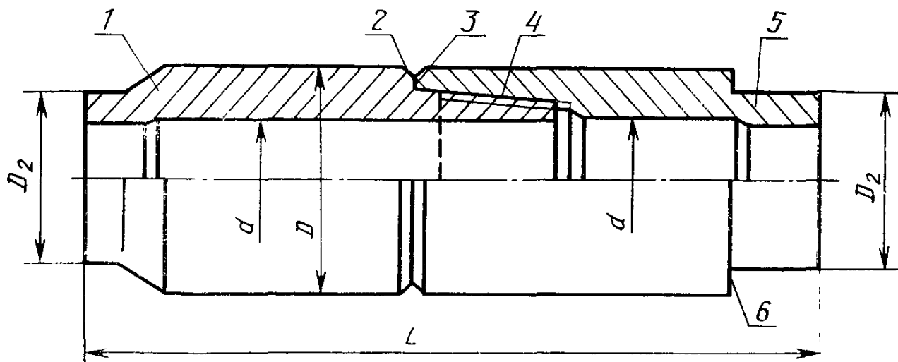
1—ниппель; 2—упорный уступ; 3—упорный торц; 4—замковая резьба; 5—муфта; D—наружный диаметр; L—длина замка в сборе; 6—заплечик под элеватор
