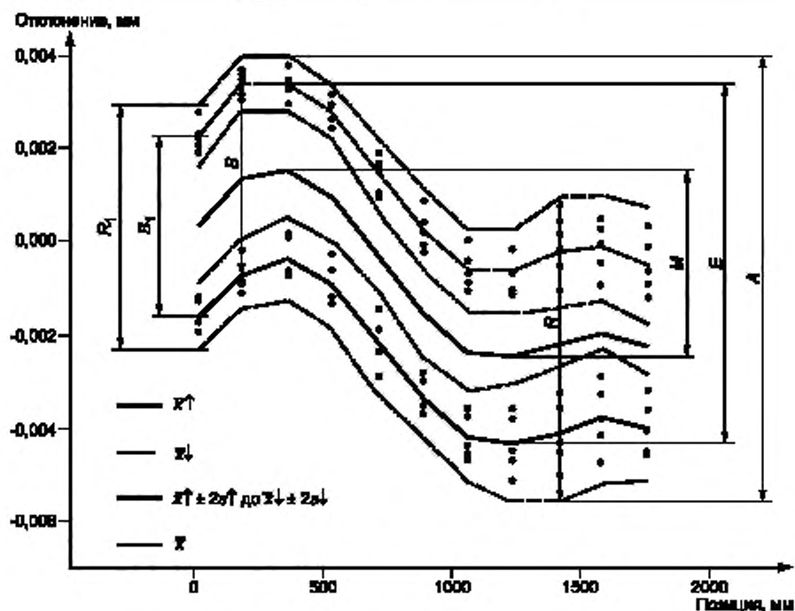
Рисунок А.1 — Точность и повторяемость двустороннего позиционирования
