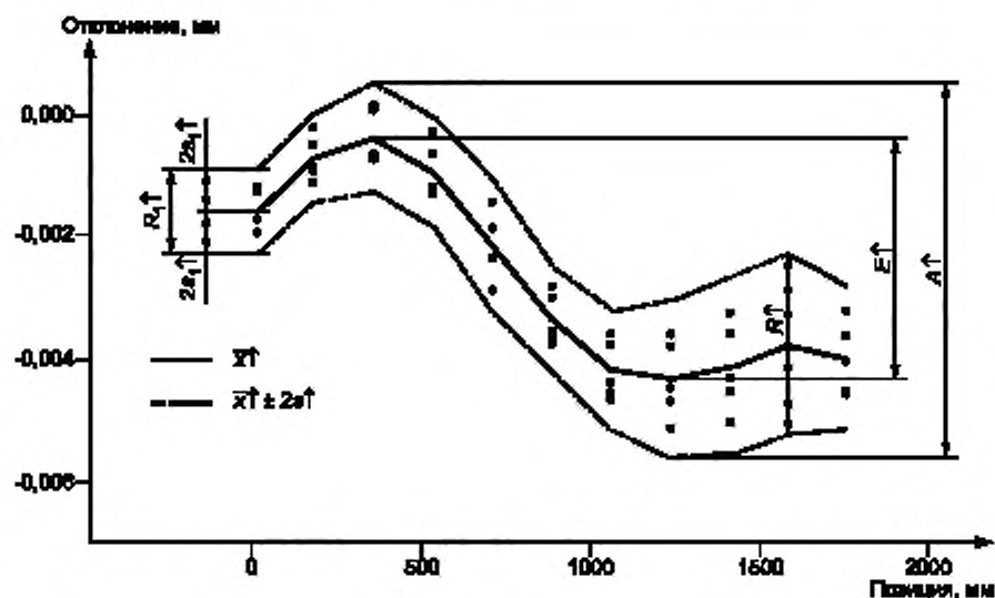
Рисунок А.2 — Точность и повторяемость одностороннего позиционирования
