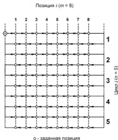
Рисунок 1 — Стандартный цикл измерений
