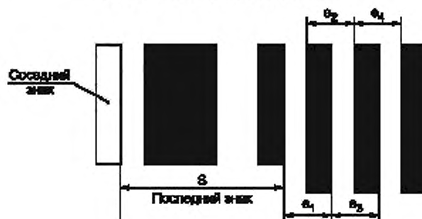
Рисунок 8 — Размеры вспомогательных шаблонов
