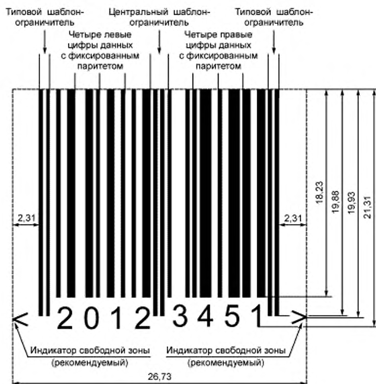
Рисунок Е.4 — Символ EAN-8
