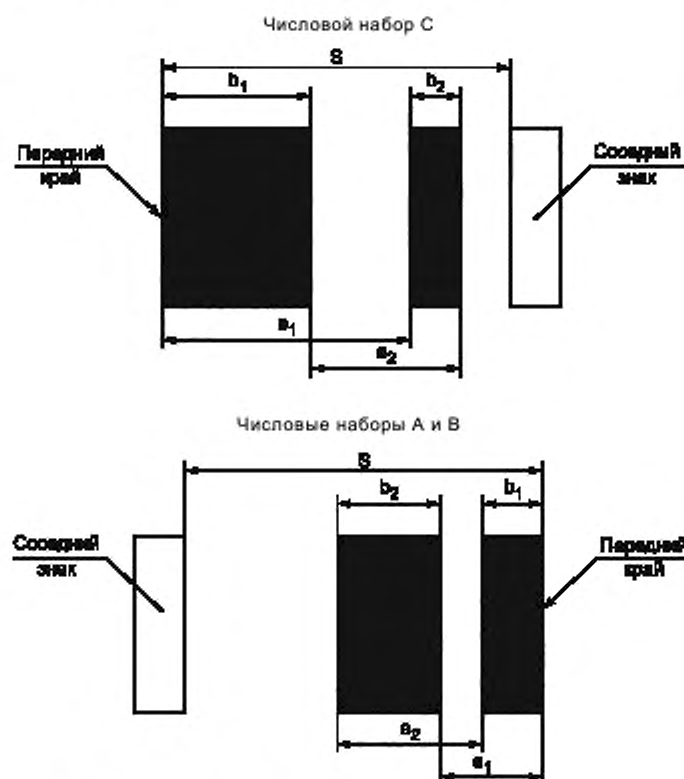
Рисунок 7 — Размеры для декодирования знаков символов
