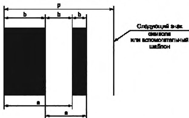
Рисунок F.1 — Размеры для определения допусков
