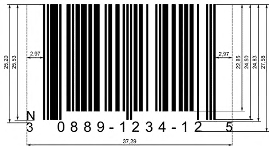
Рисунок Е.3 — Примеры вариантов исполнения символа UPC-A
