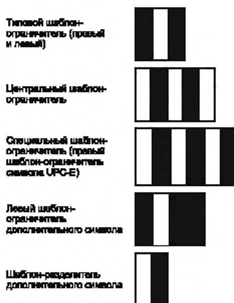
Рисунок D.2 — Представление вспомогательных шаблонов
