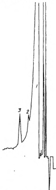
1—пропилен; 2—изобу- тан; 3—н-бутан
