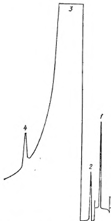
1—метан, 2—этан; 3—этилен; 4—пропан
