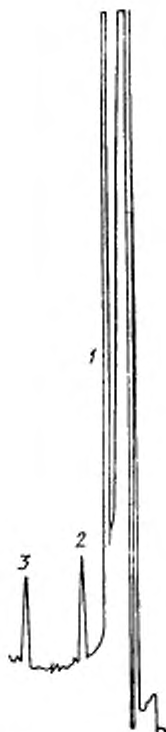
1—этилен; 2—пропадиен; 3—бутадиен 1,3
