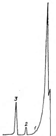
1—кислород; 2—азот; 3—метан
