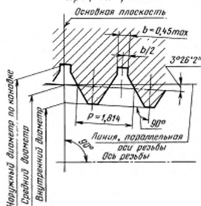
Профиль резьбы
