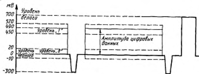
Рисунок 2 — Уровни сигнала цифровых данных сигнала телетекста
