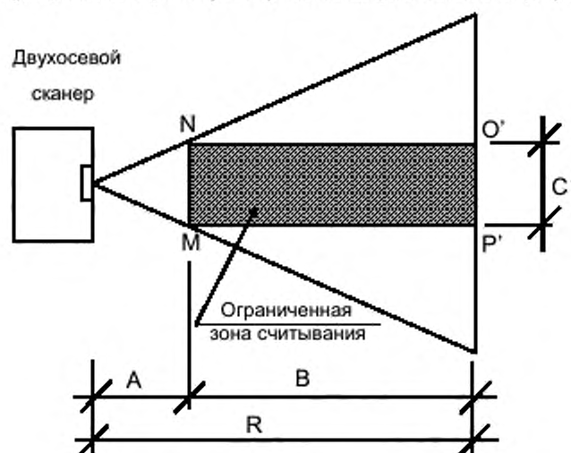
Рисунок 3 – Пример ограниченной зоны считывания (зона MNO'P')
