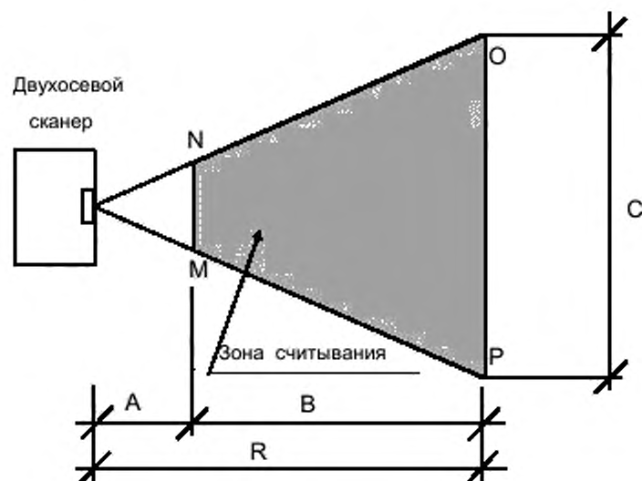
Рисунок 2 – Пример зоны считывания (зона MNOP)
